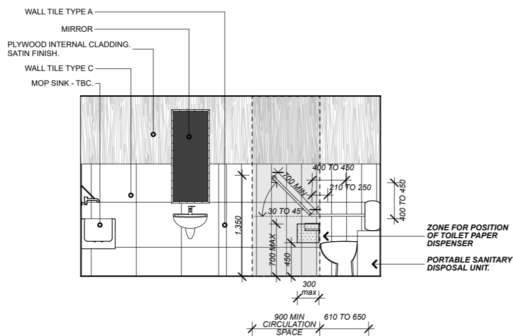
PWD 2 1:50
